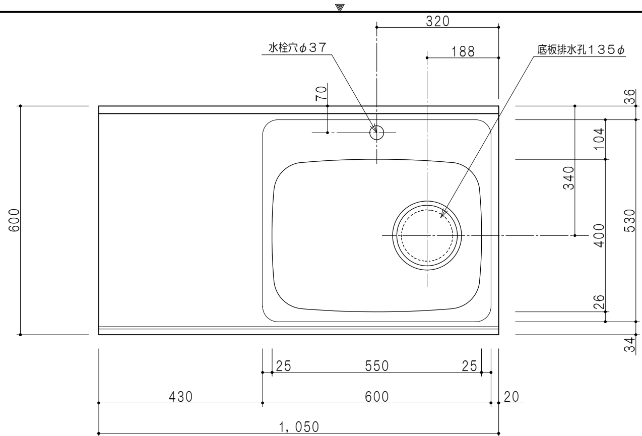
平面図
