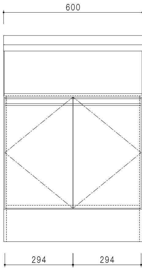
平面図
