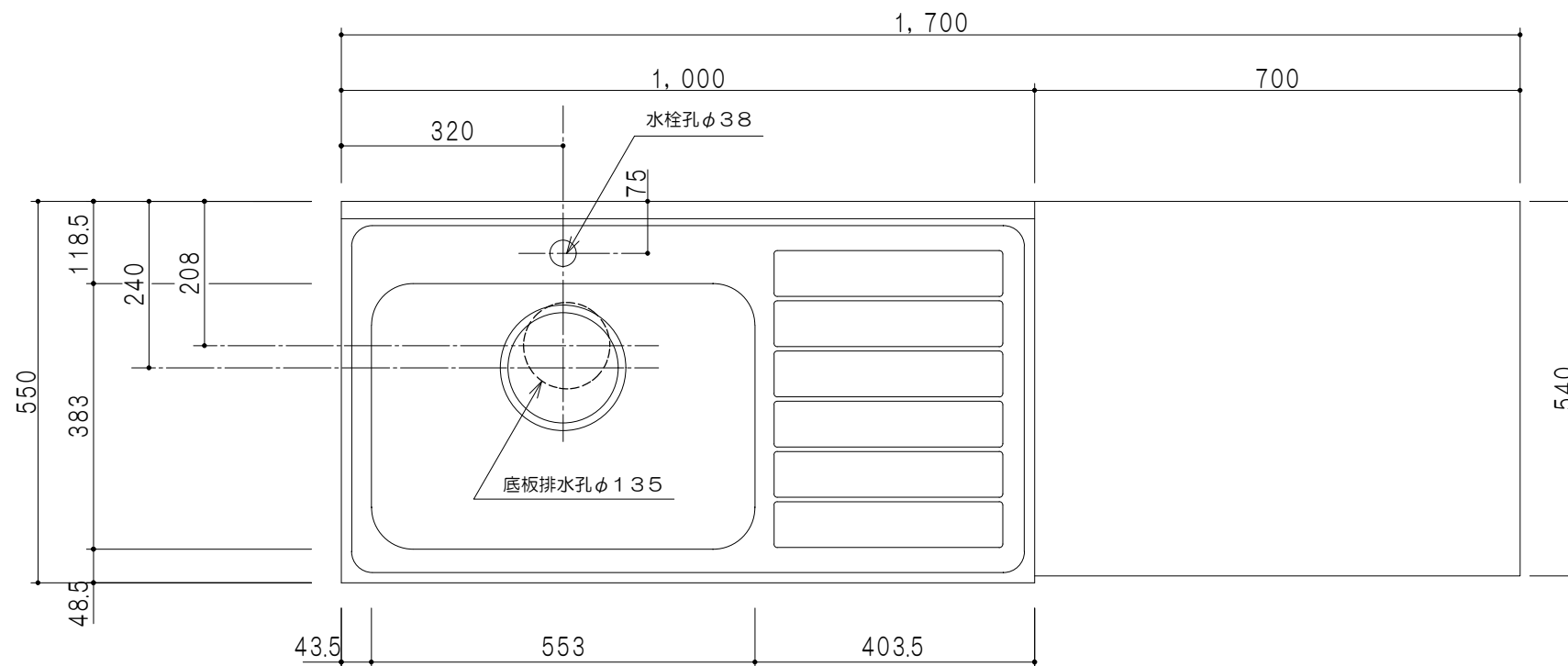
平面図
