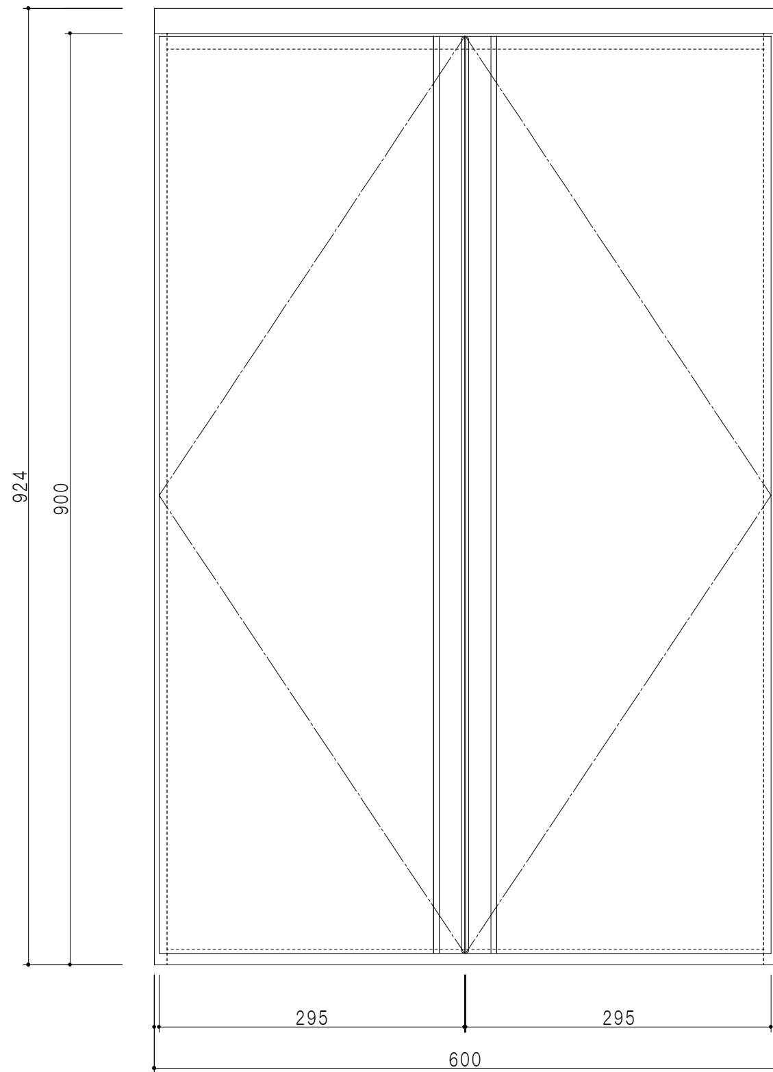
立面図
