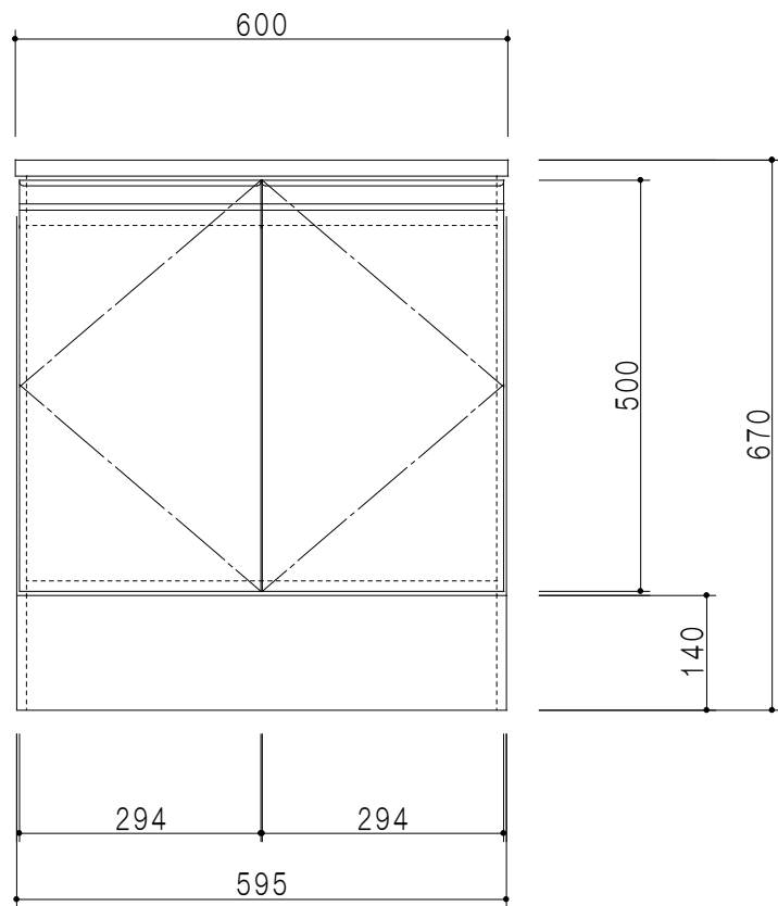
立面図
