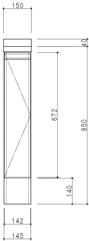
立面図
