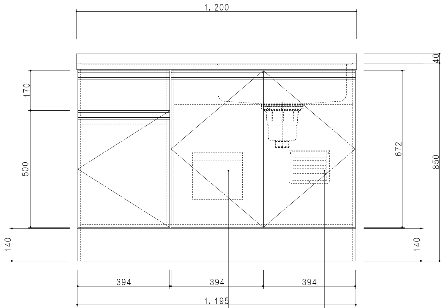
立面図
