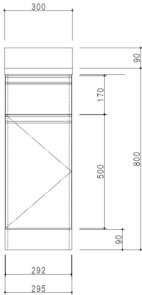
立面図
