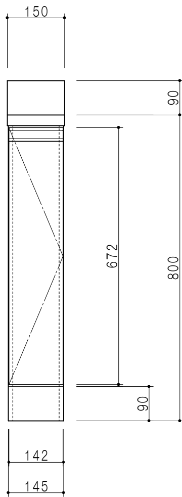
立面図
