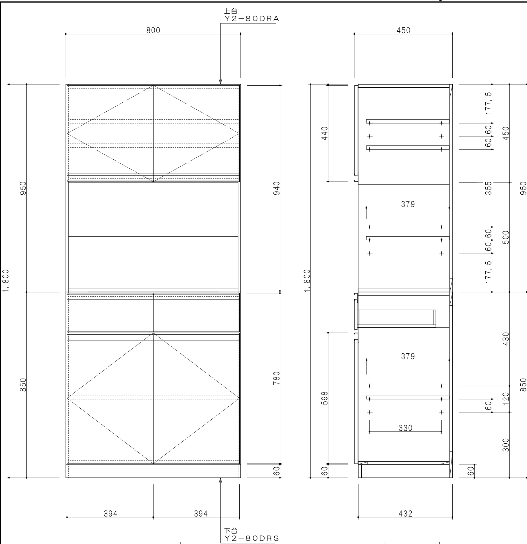
立面図
