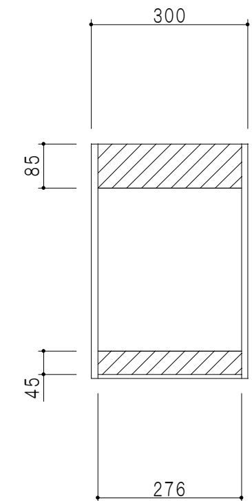
背面図
