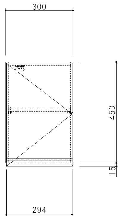
立面図
