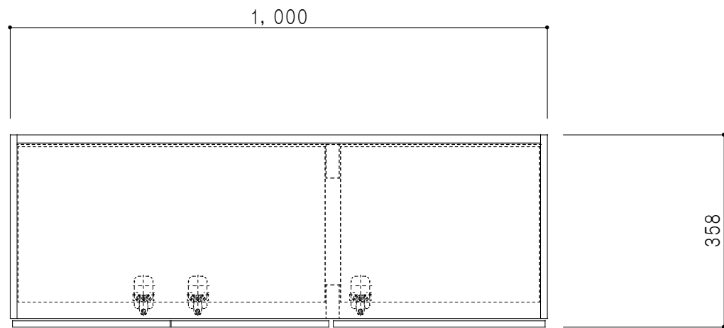
平面図
