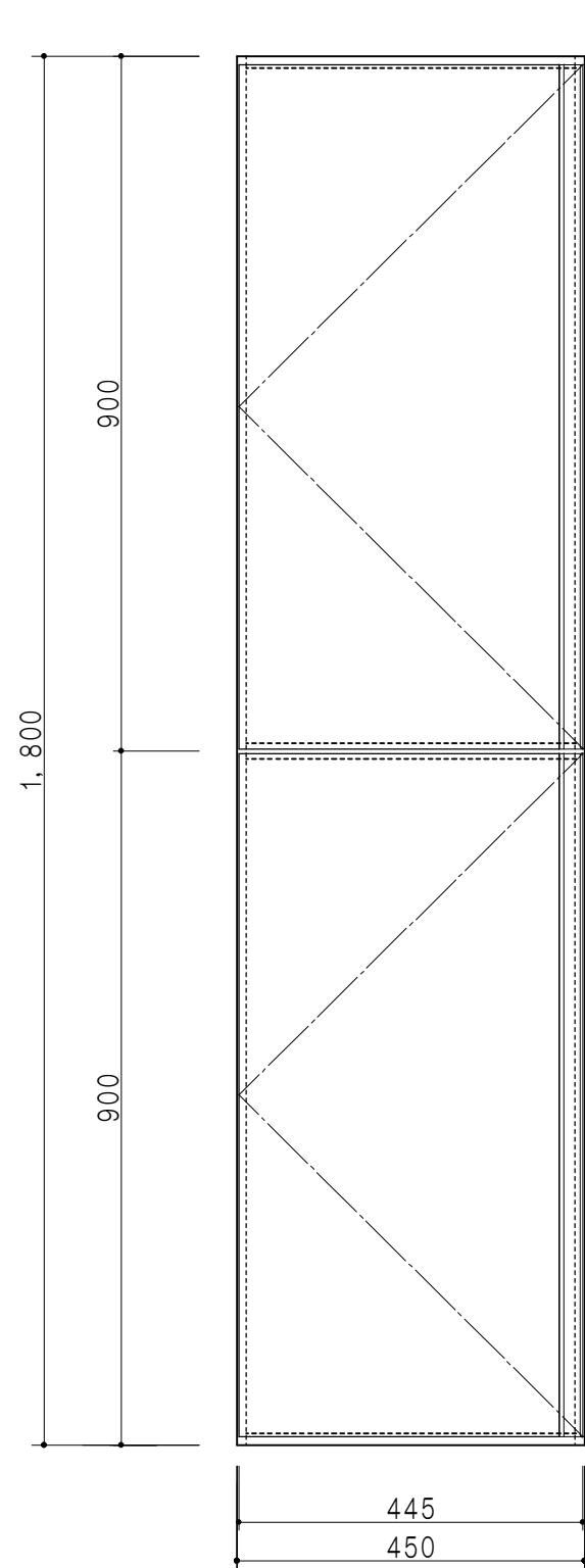
立面図
