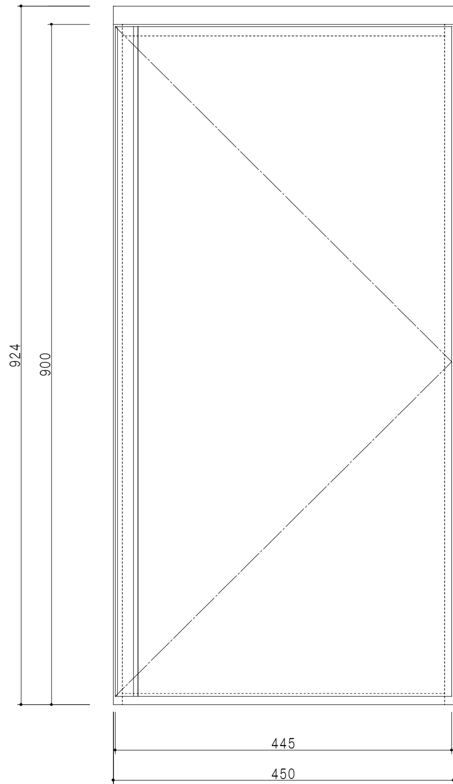
立面図
