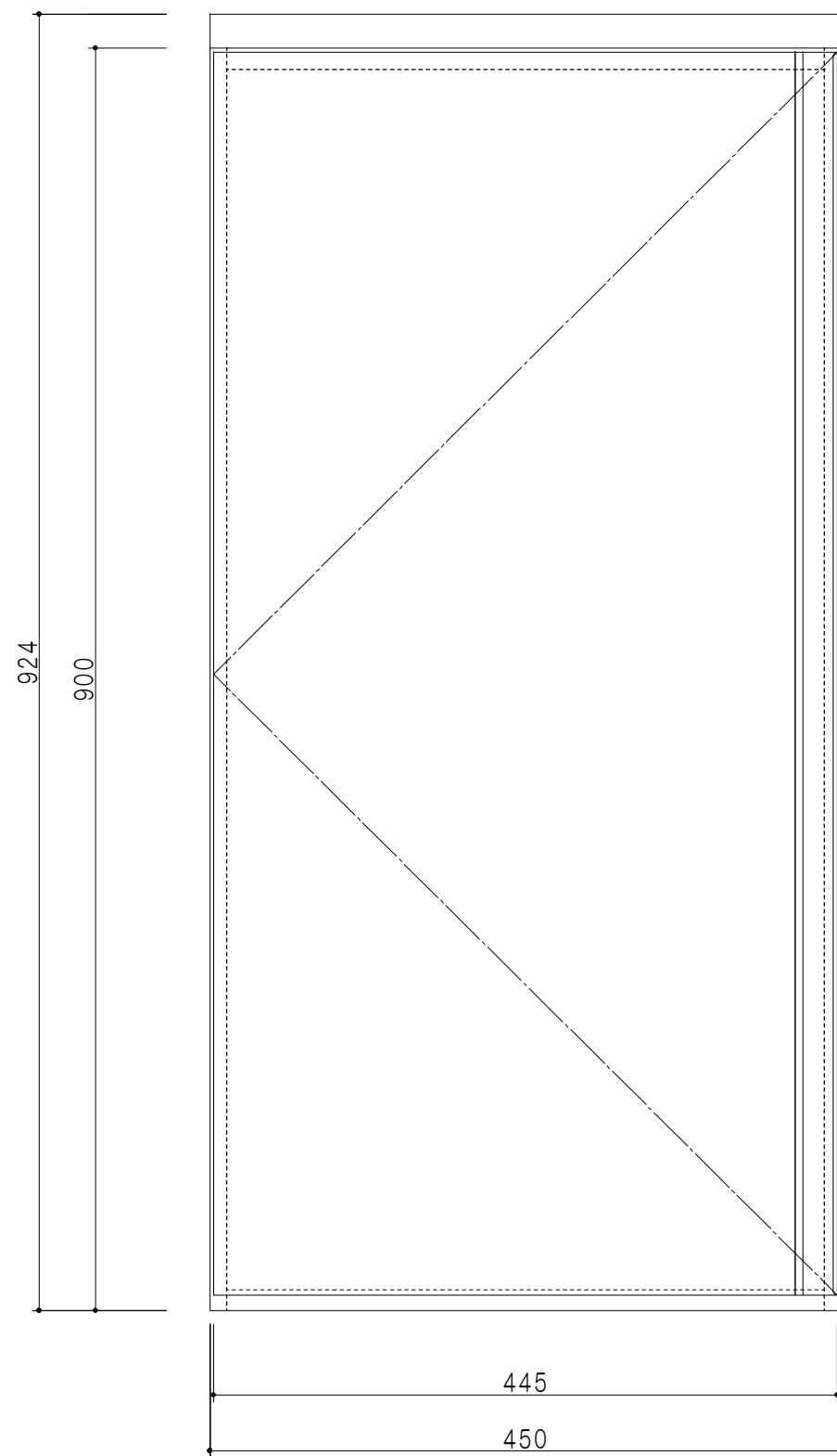
立面図
