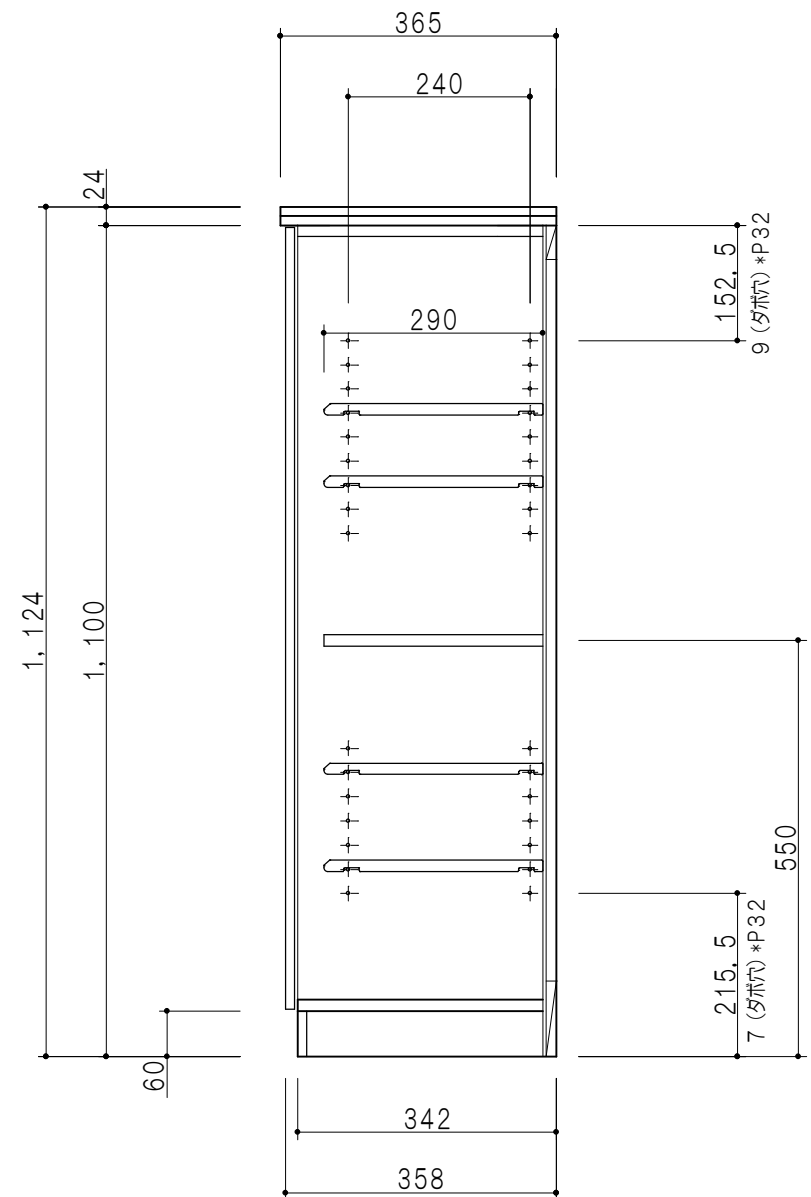
断面図
