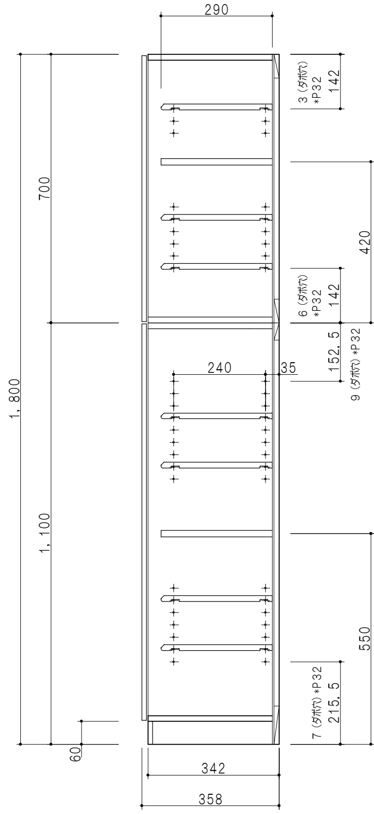
断面図
