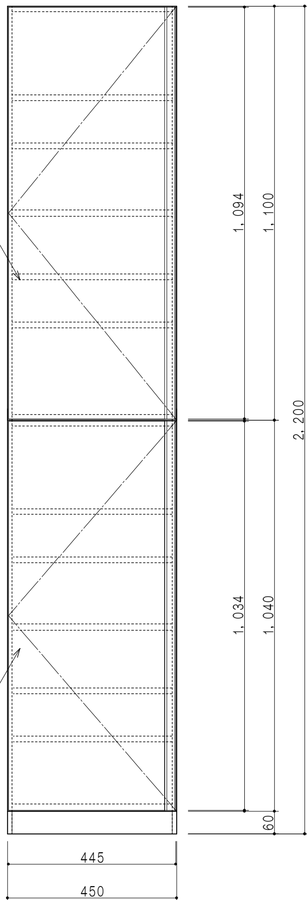
立面図
