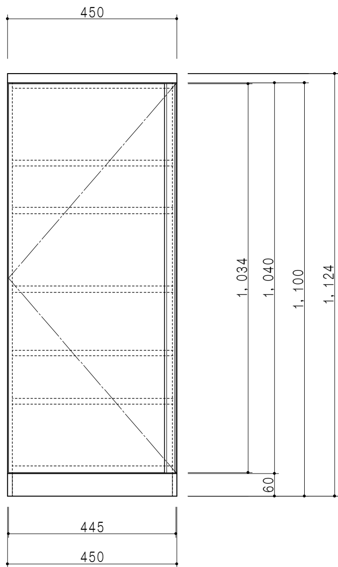
立面図
