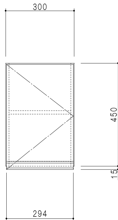
立面図
