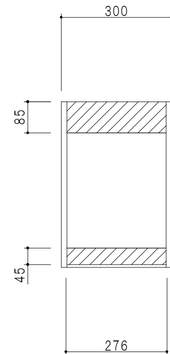
背面図
