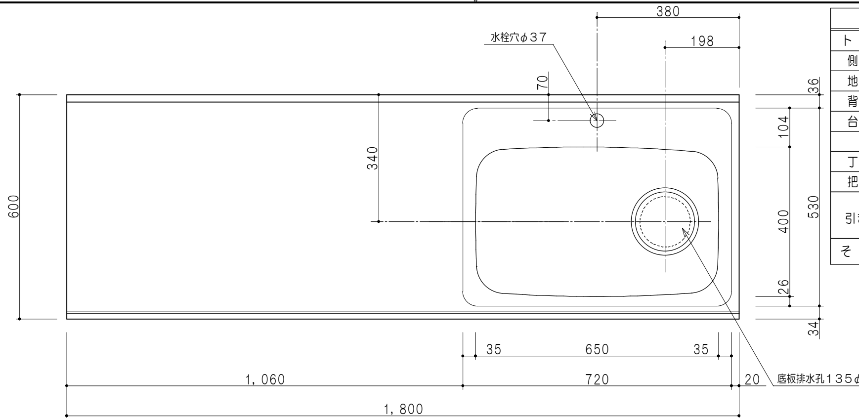
平面図
