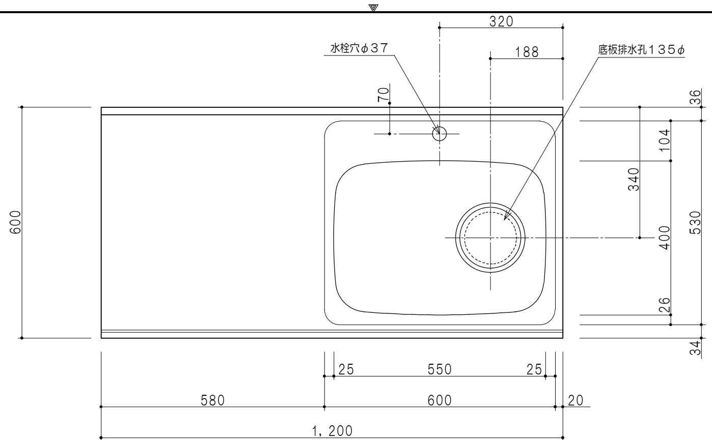
平面図
