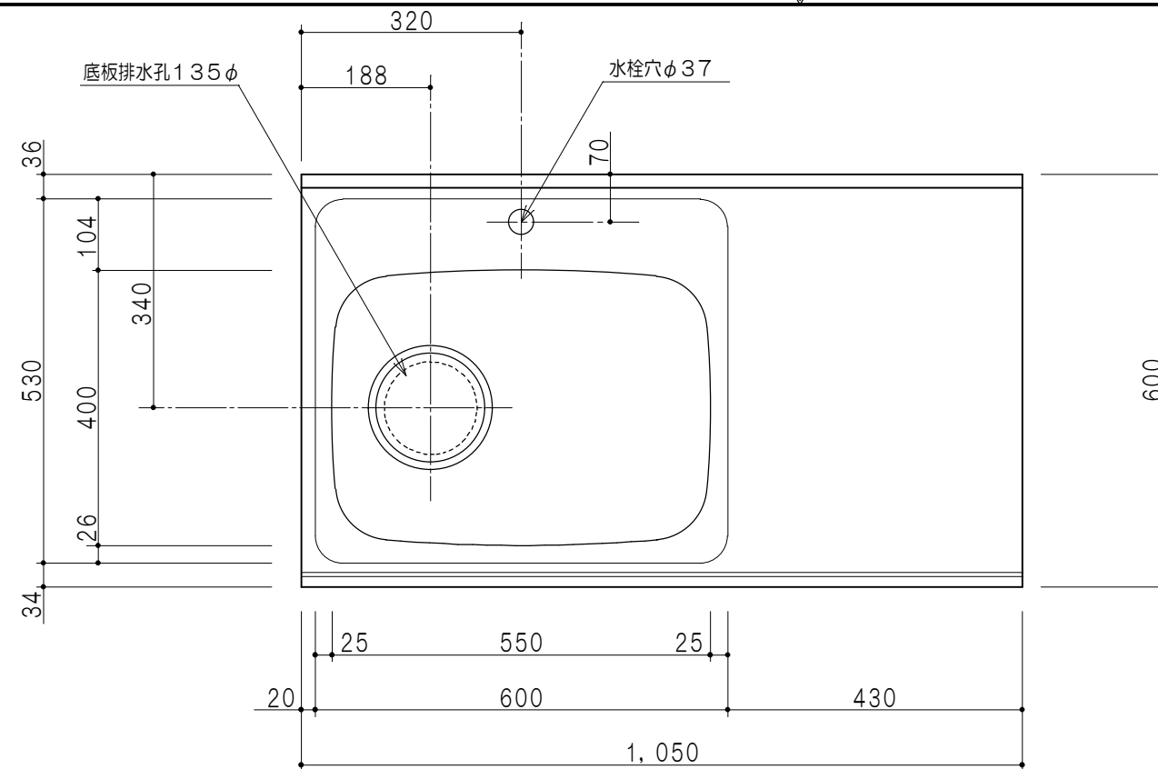
平面図
