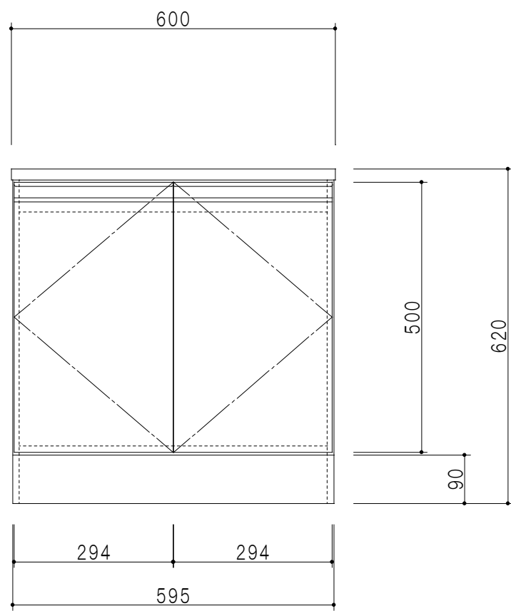
立面図
