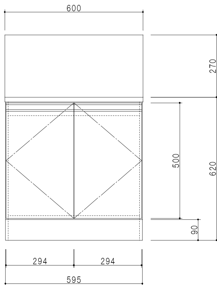
立面図
