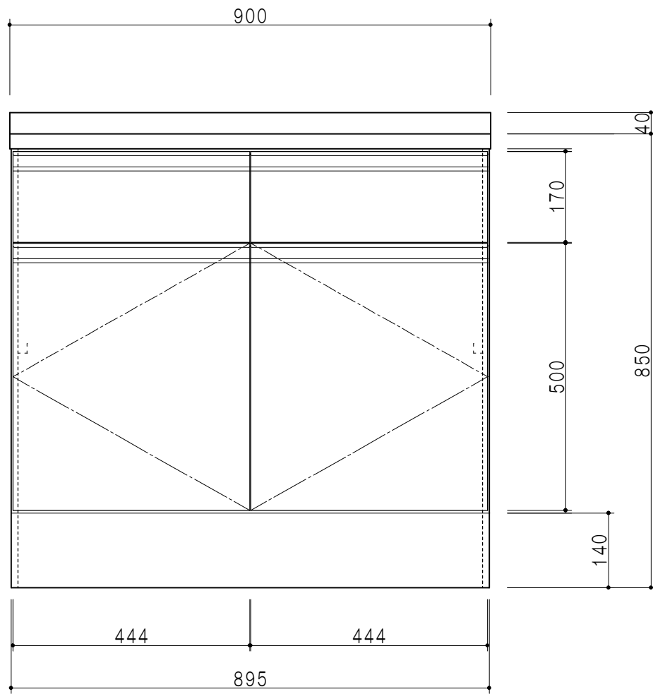
立面図
