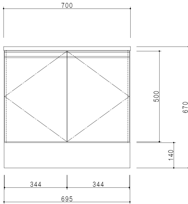
立面図
