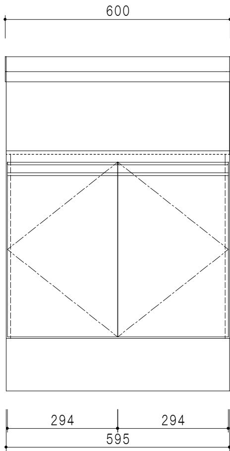
立面図
