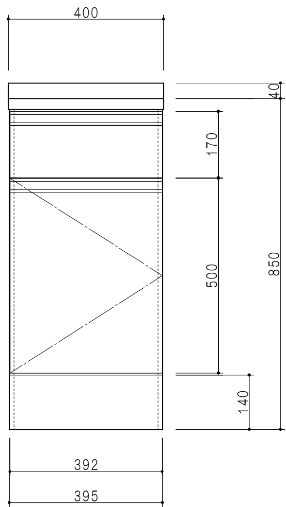
立面図
