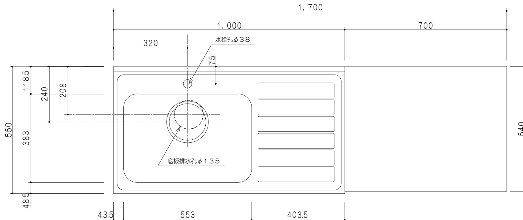
平面図
