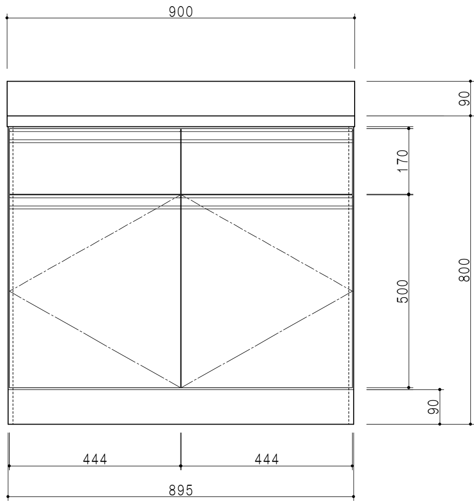
立面図
