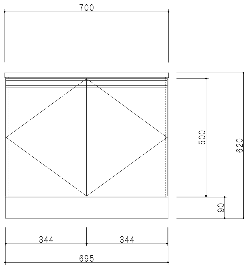
立面図
