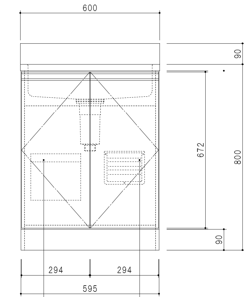
立面図
