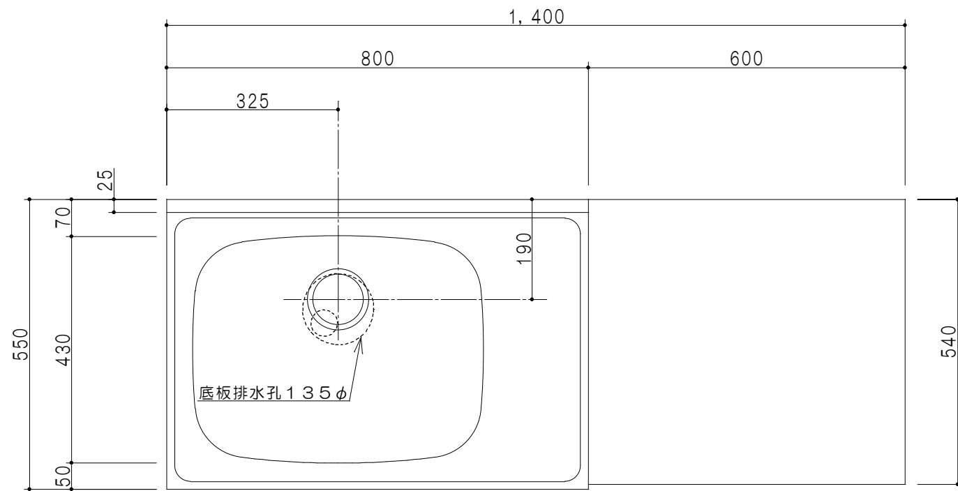
平面図
