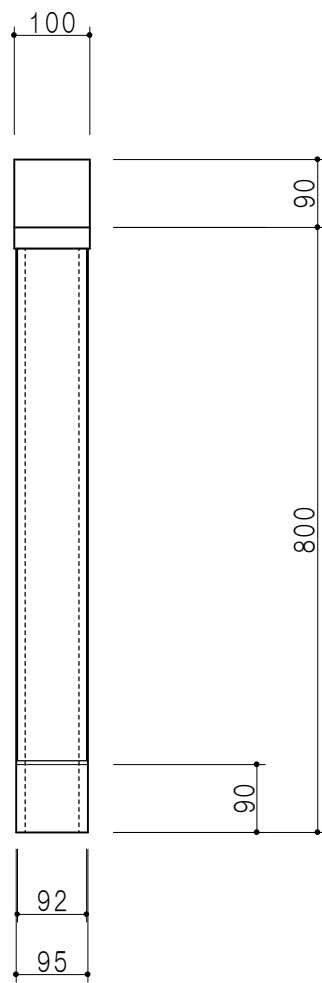
立面図
