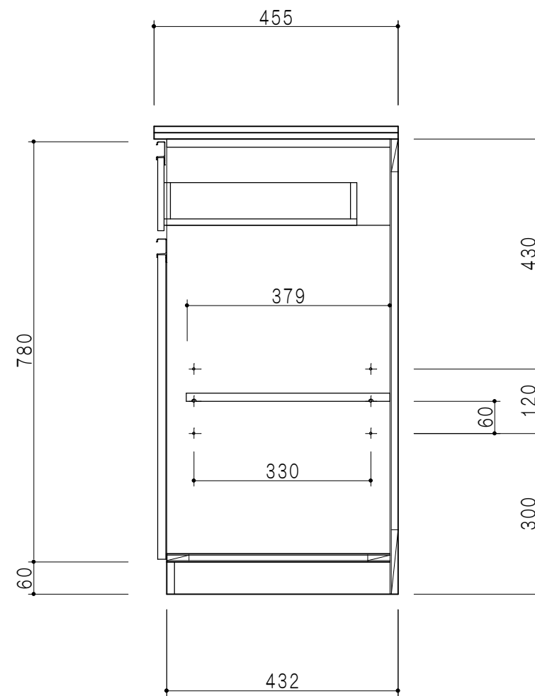
断面図
