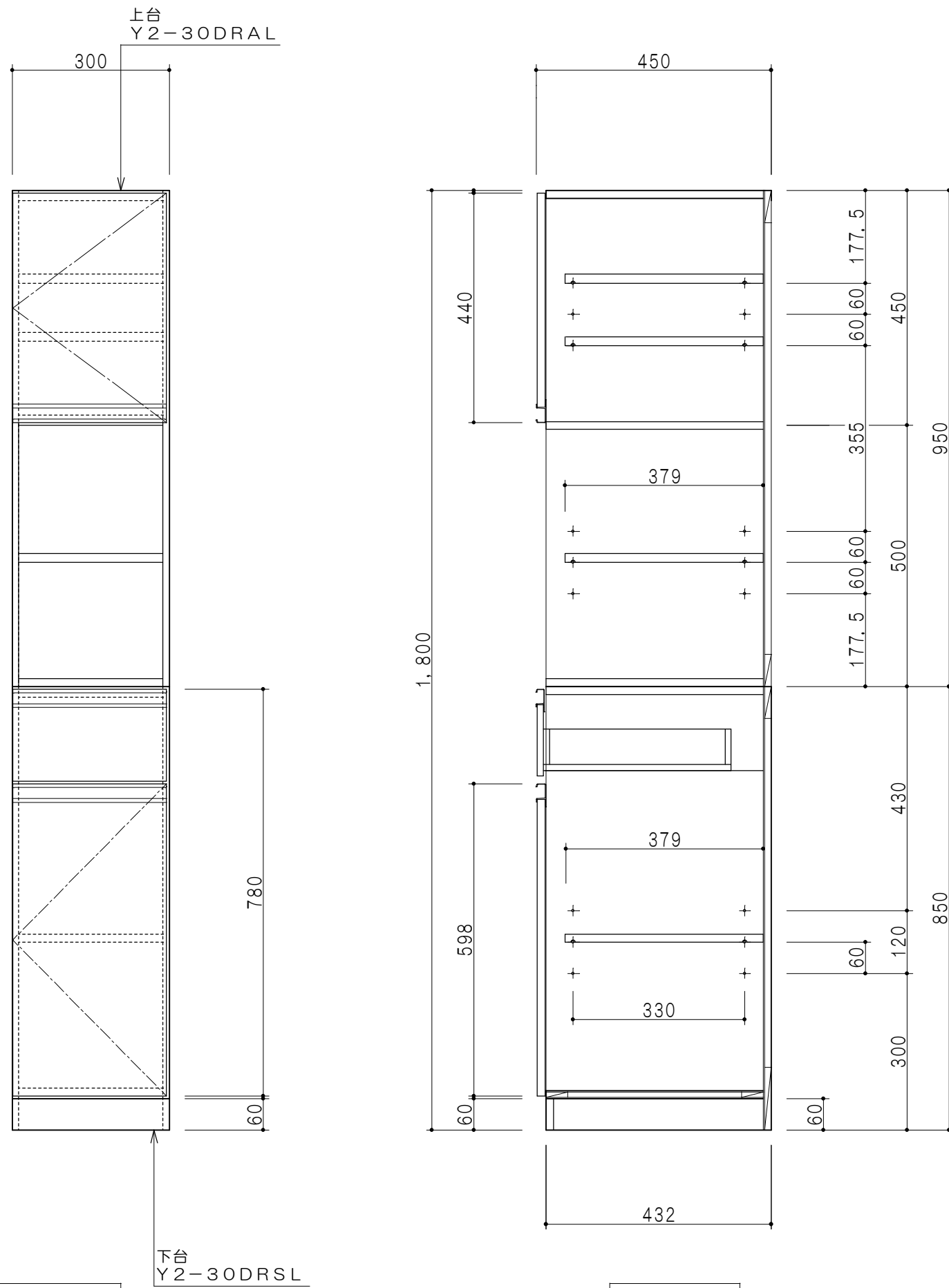
立面図
