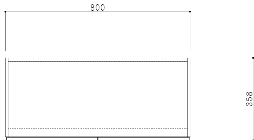
平面図
