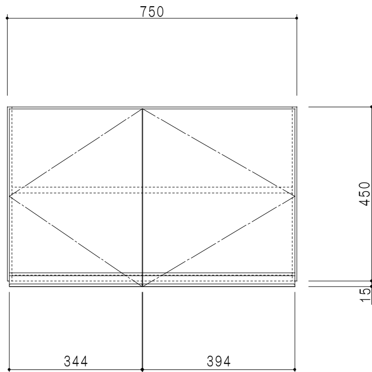
立面図
