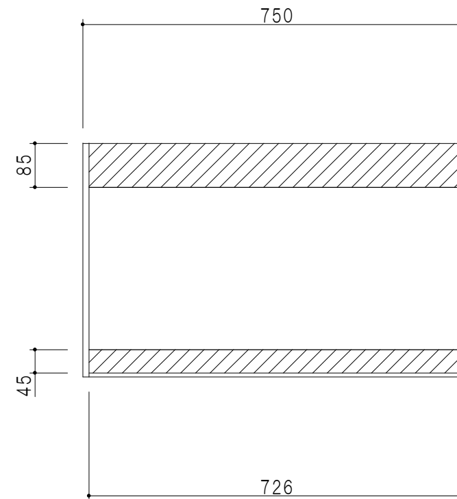
背面図
