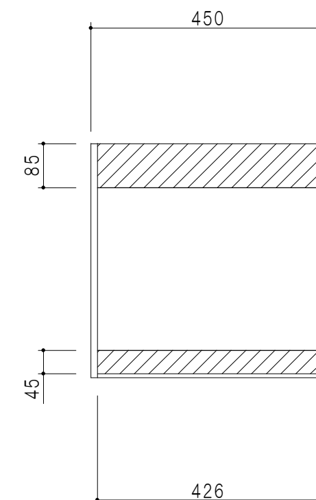
背面図
