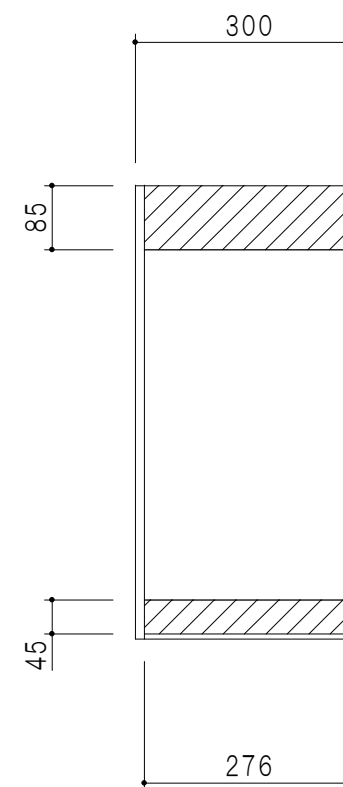
背面図
