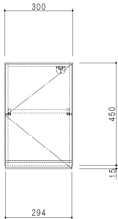
立面図
