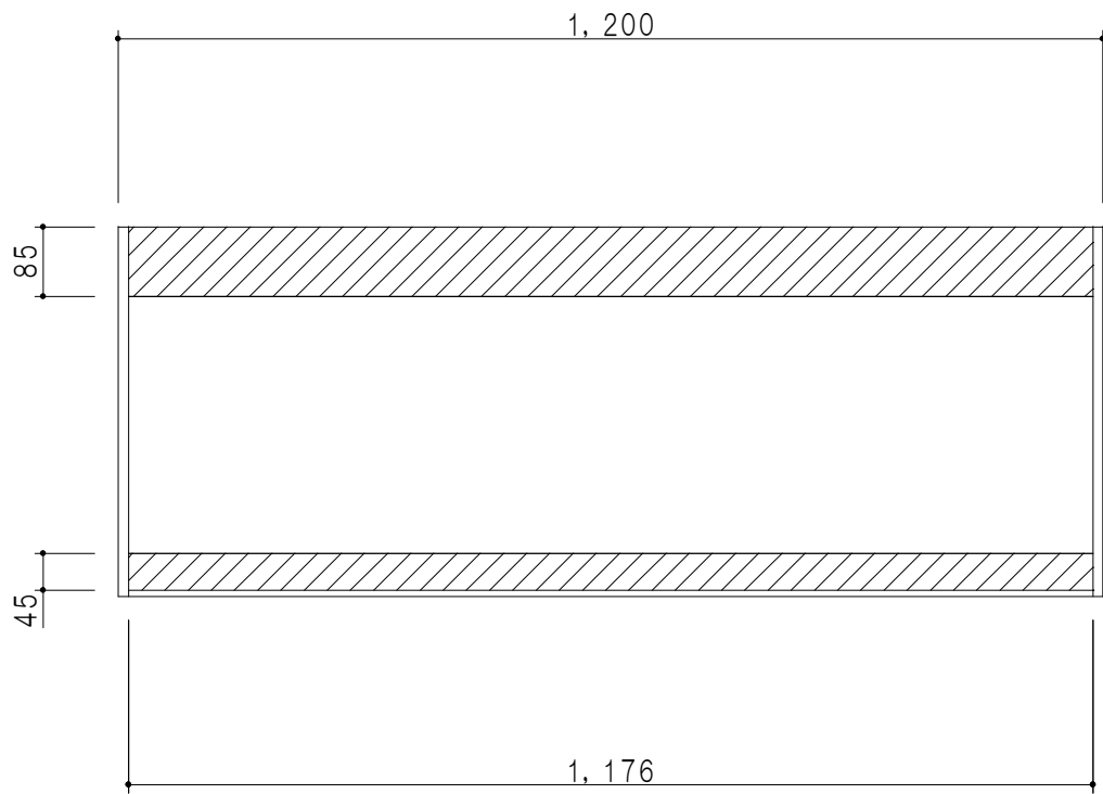
背面図
