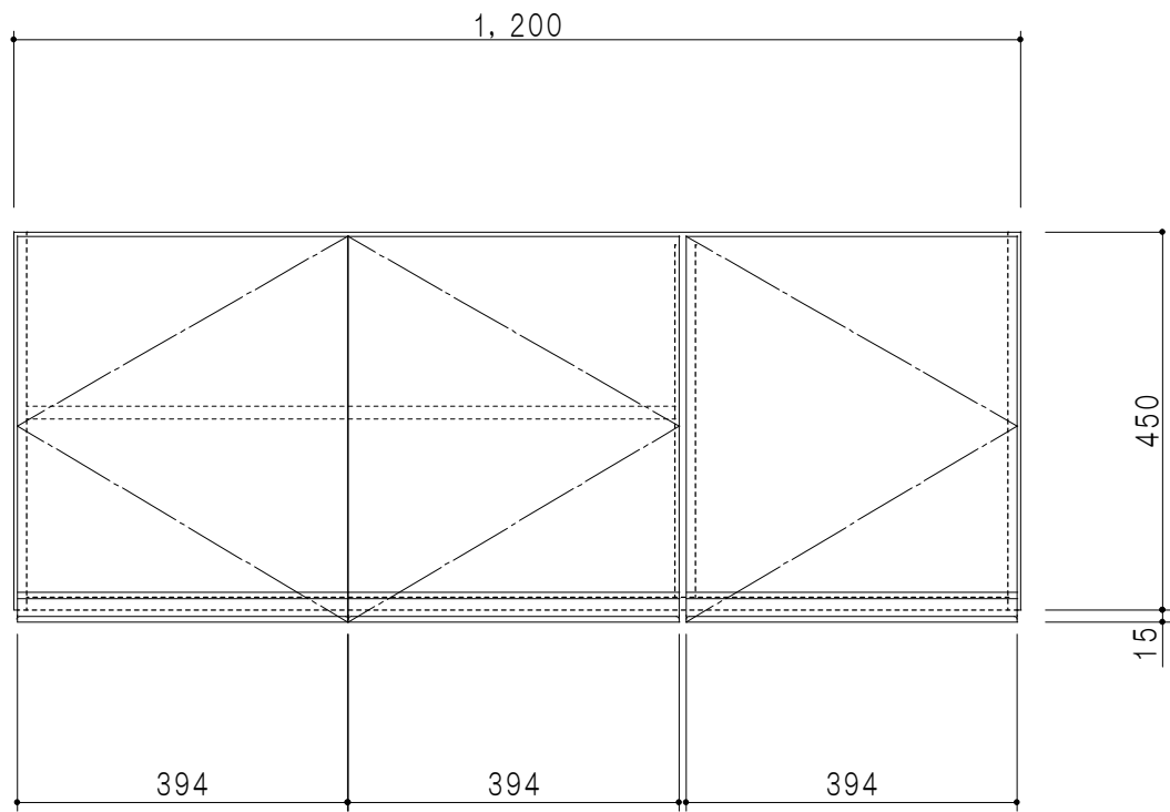
立面図
