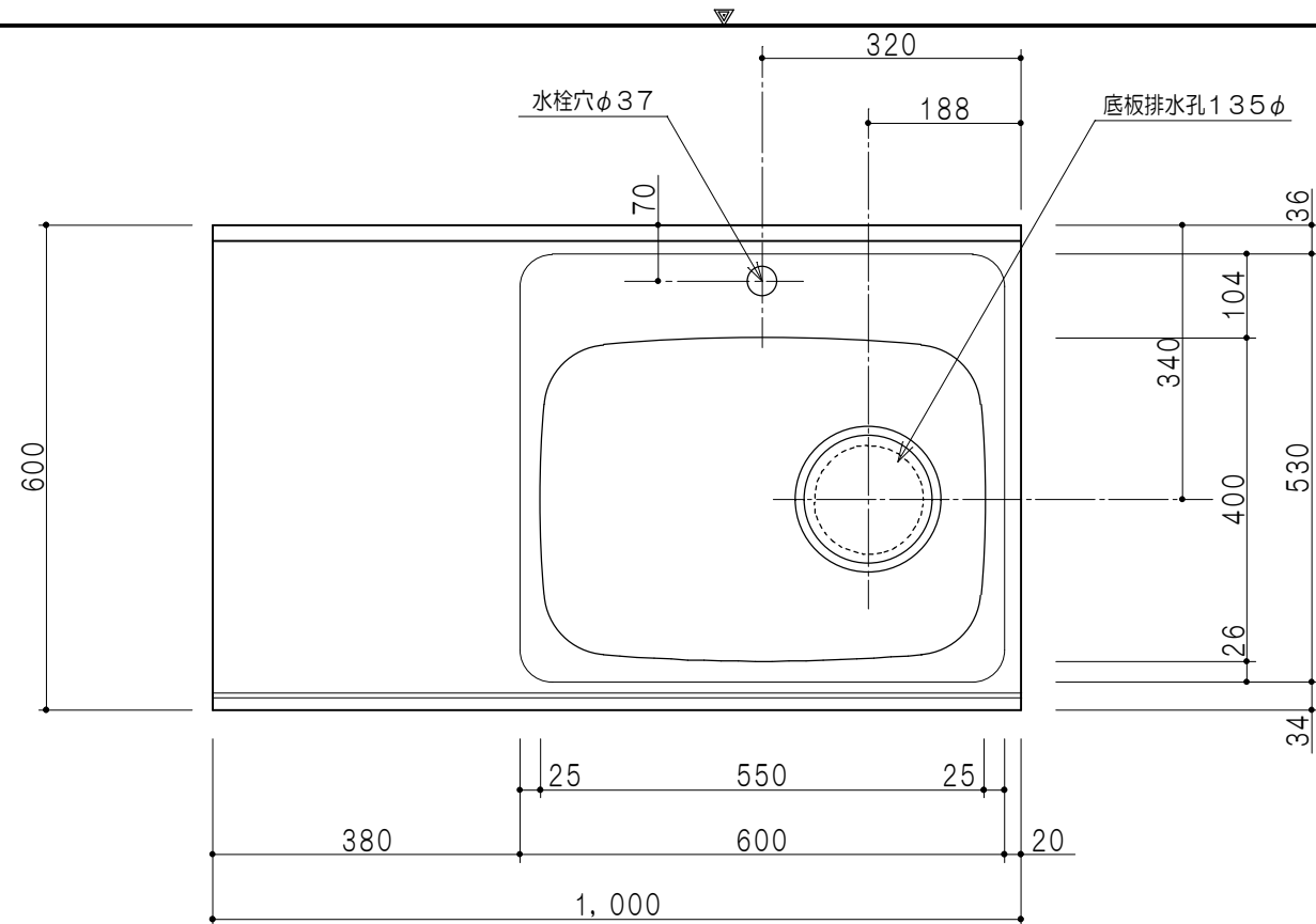
平面図
