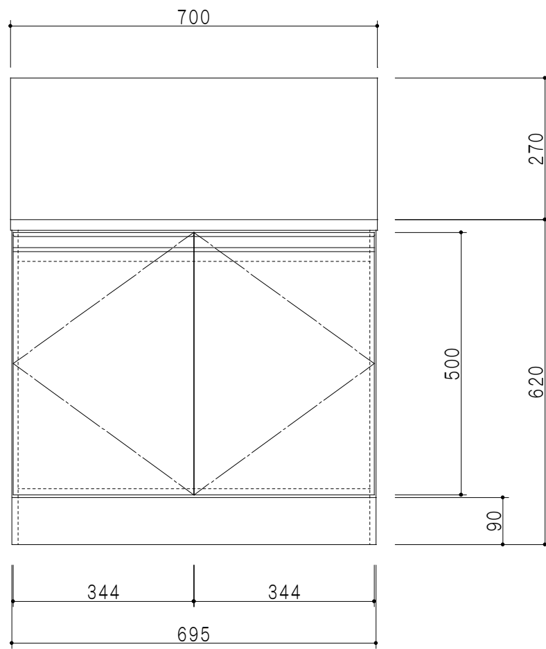
立面図
