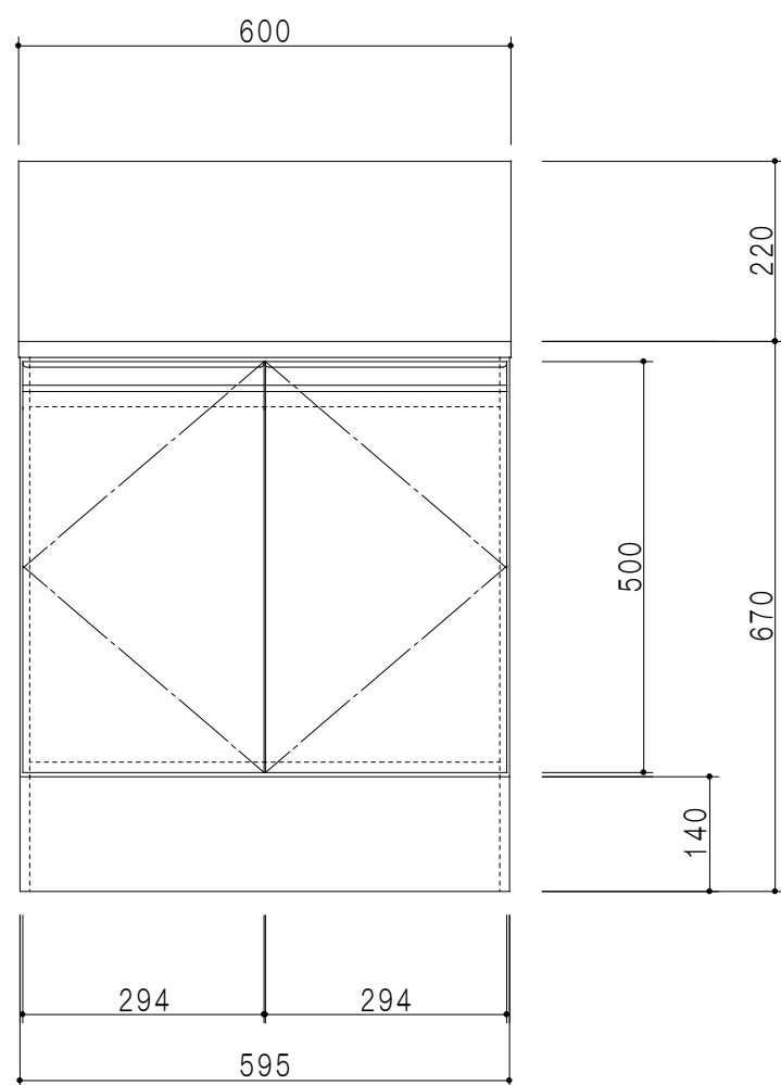
立面図
